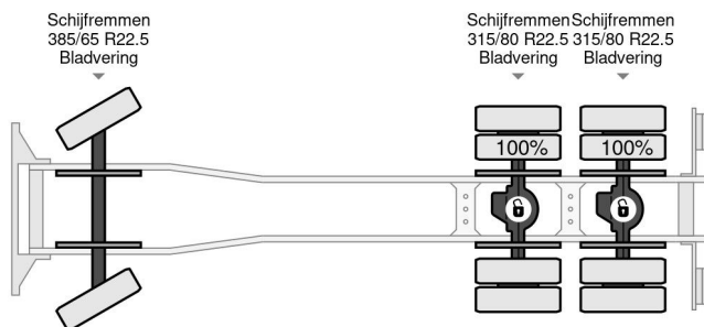
DAF CF 480 FAT + Crane FASSI F235A.2.23 E-DYNAM... 6x4
