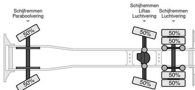
DAF CF 330 FAG as-tronic 6*2 + VDK PUSHER IIK/IID ... 6x2 Referentienummer: HVW-1166 - 1YFN958 - 0G052654
