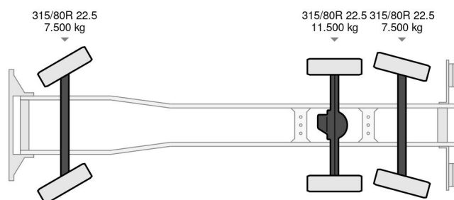
DAF CF 75 250 FAN + Geesink garbage + Krane HIAB 195 6x2
