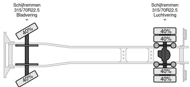
Mercedes-Benz ANTOS 1924
