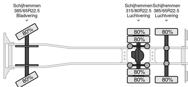
Mercedes-Benz ANTOS 2843
