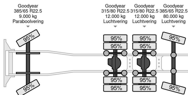
DAF CF 480 FAW 8x4 +container hook WAF 22T + crane H...
